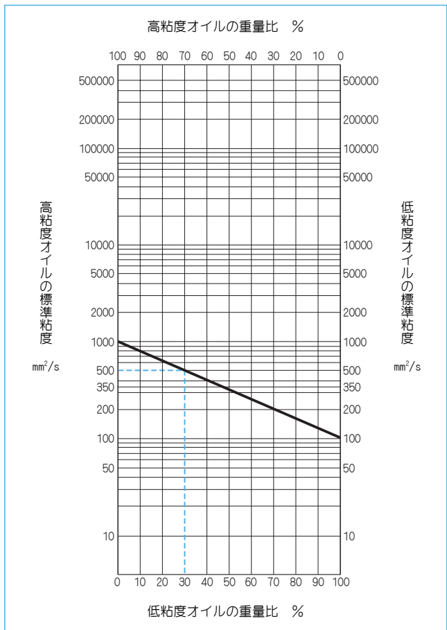
図7 シリコンオイルの混合チャート
